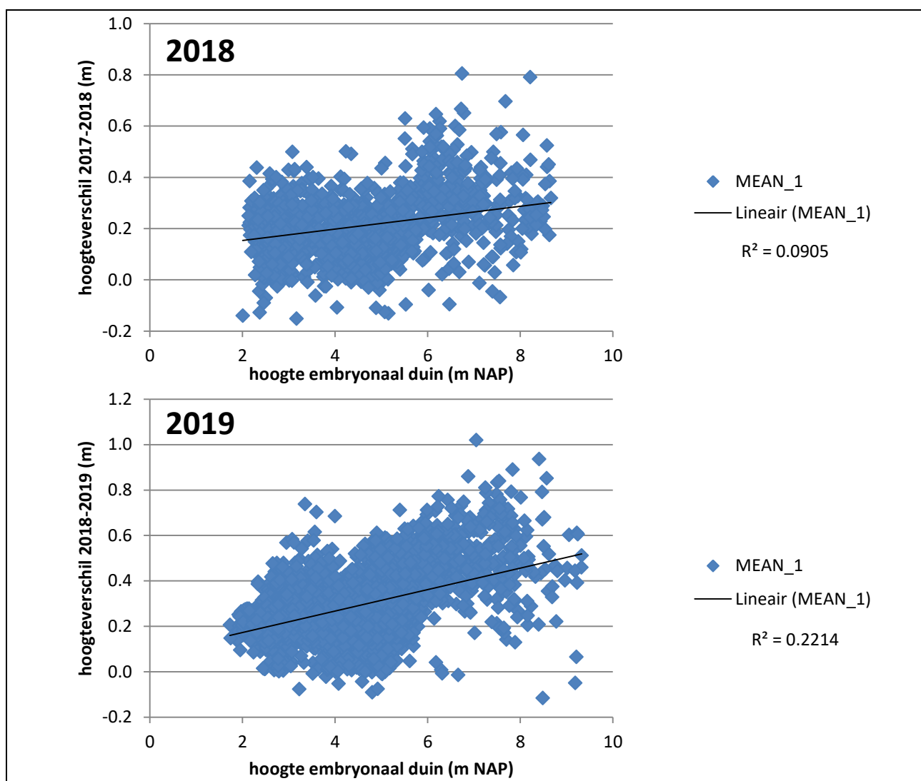
Figuur 14. Correlatie tussen hoogte van de embryonale duinen (in m NAP) en hoogteverschil tussen respectievelijk 2017-2018 (boven) en 2018-2019 (onder). Het hoogteverschil is steeds bepaald tussen de RWS opname van de Zandmotor en de Shore opname van het jaar daarna.
