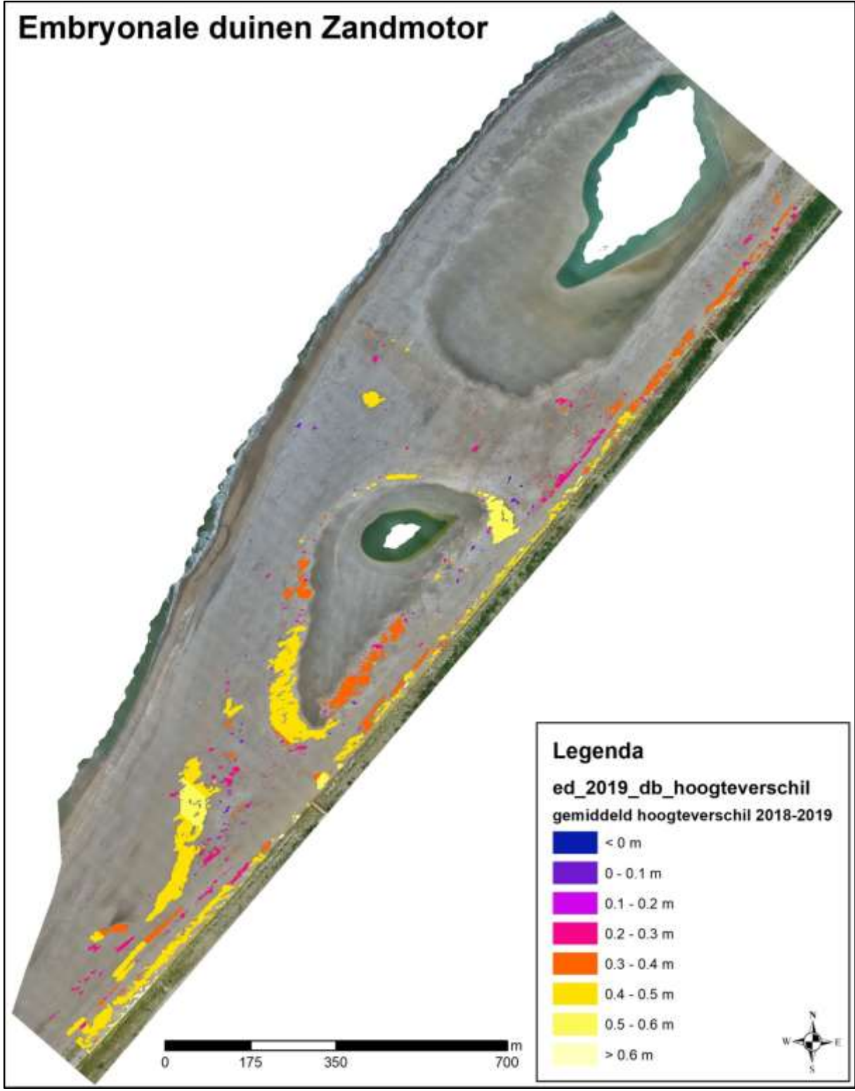
Figuur 10. Gemiddeld hoogteverschil per duinvlak tussen 2018 (RWS opname Zandmotor)-2019 (Shore).
