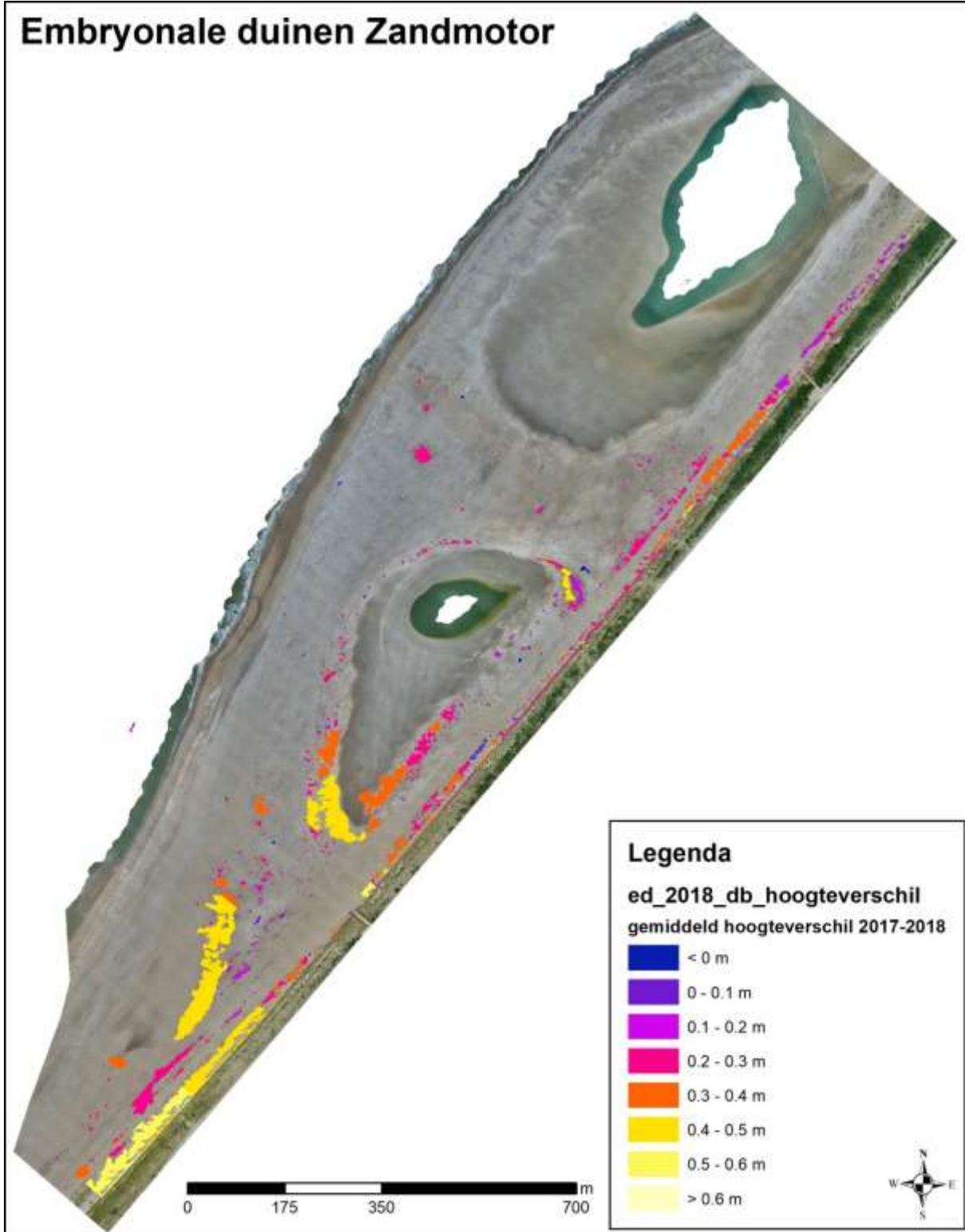
Figuur 9. Gemiddeld hoogteverschil per duinvlak tussen 2017 (RWS opname Zandmotor)-2018 (Shore).
